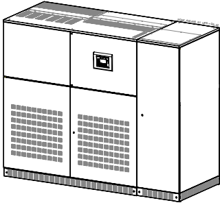
Рис. 10.5.2-1 Расположение шкафов
