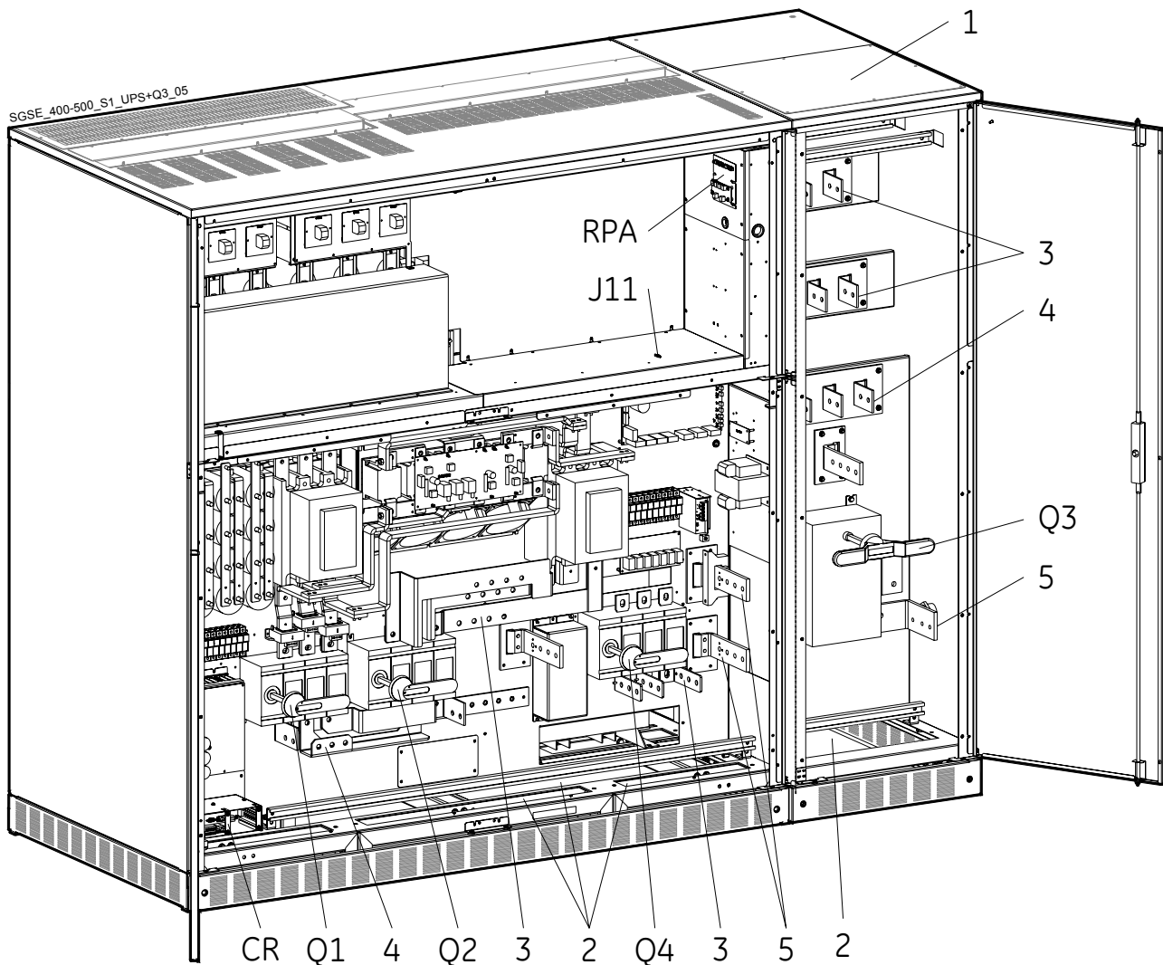
Рис. 2.2-6 Общий вид со снятыми защитными панелями
