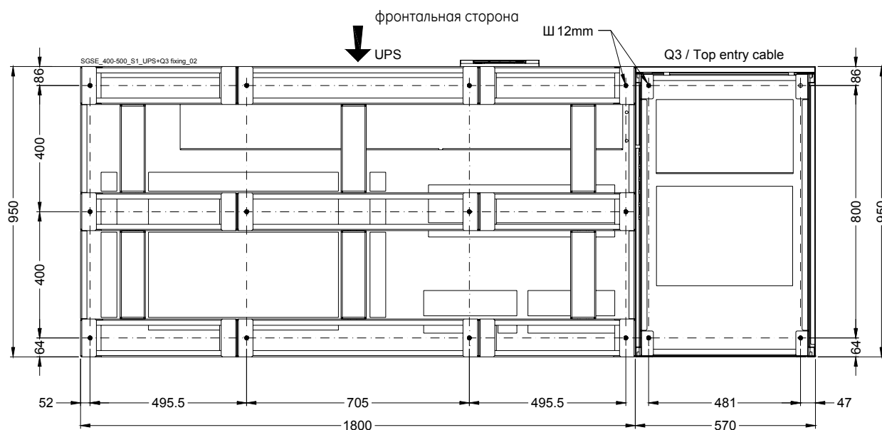
Рис. 5.4.1-5 SG-CE Series 400-500 кВА с опциональным шкафом выключателя АКБ Q3 и/или ввода кабелей сверху – Точки крепления ИБП к полу (вид на корпус ИБП снизу)
