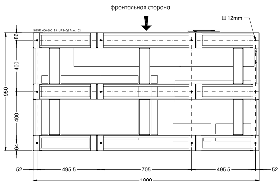
Рис. 5.4.1-5 SG-CE Series 400-500 кВА – Точки крепления ИБП к полу (вид на корпус ИБП снизу)
