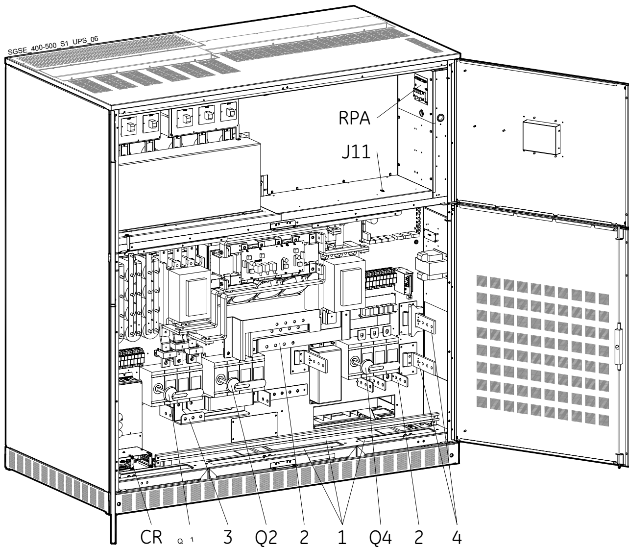
Рис. 2.1-6 Общий вид со снятыми защитными панелями
