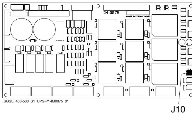
Рис. 5.6-3 P1 – плата силового интерфейса
