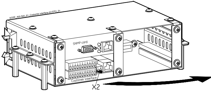
Рис. 9.1.5-1 клеммник X2 для подключения EPO
