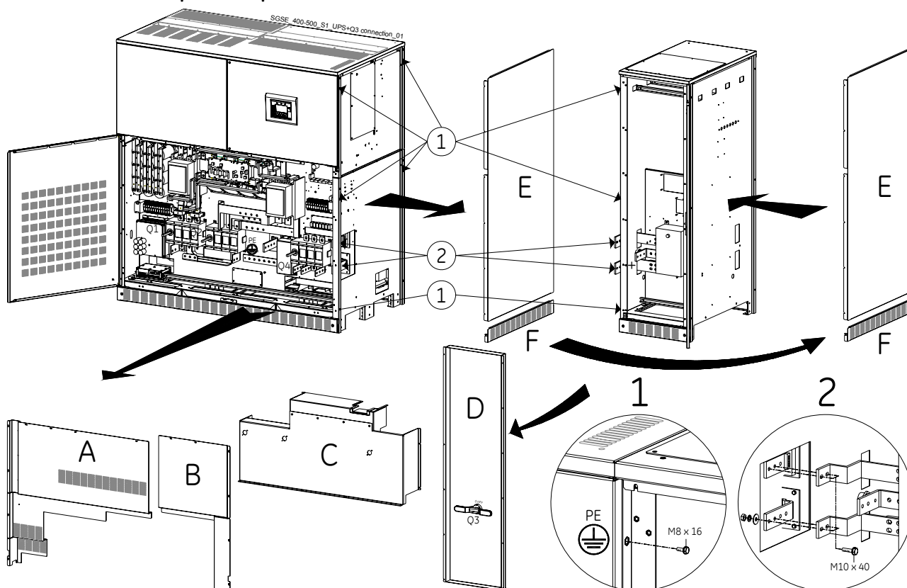
Рис. 10.5.1-2 Расстановка и сборка шкафов
