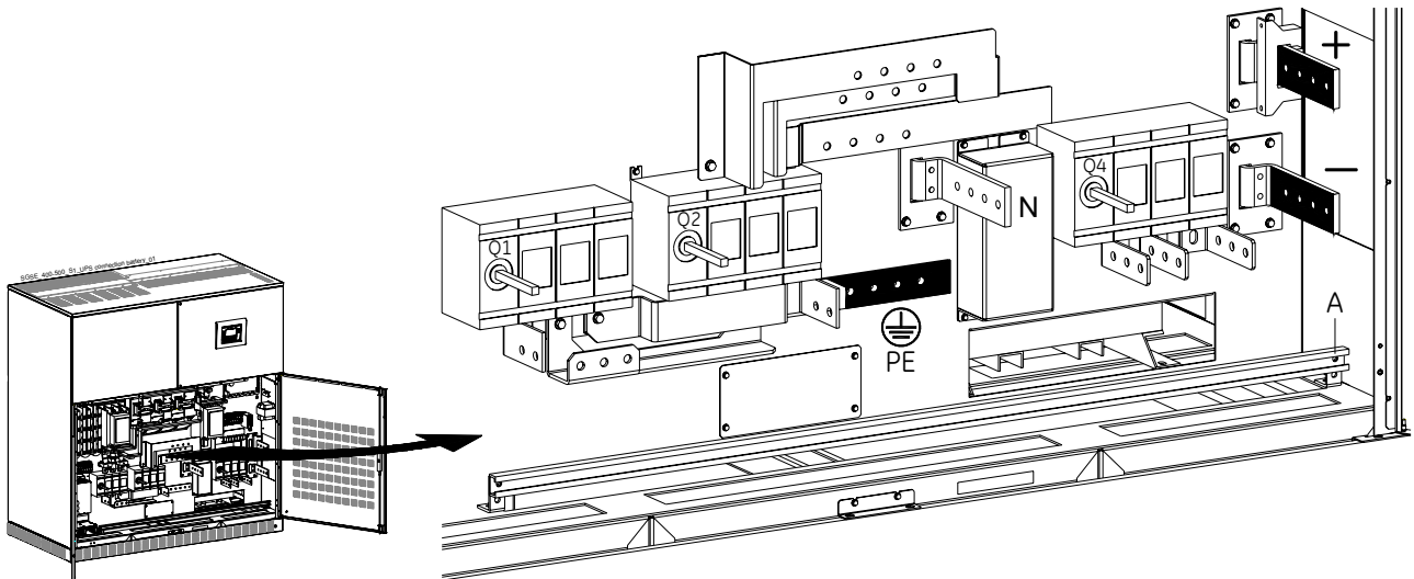
Рис. 5.8.5-1 Подключение батареи
