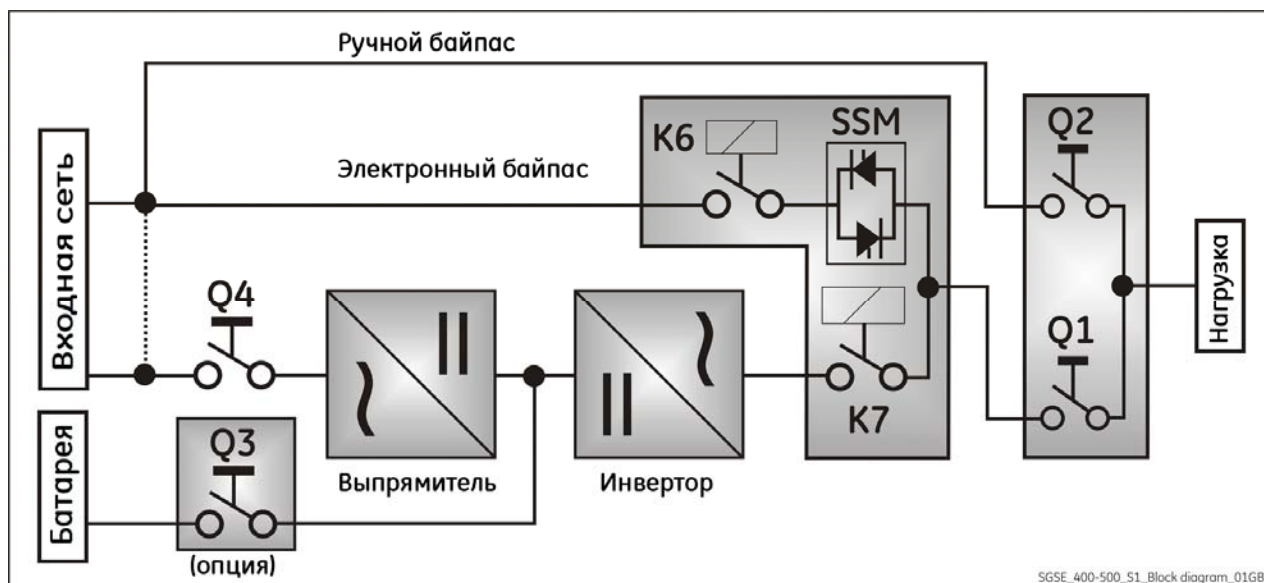
Рис. 4.1-1 Блок-схема ИБП.
