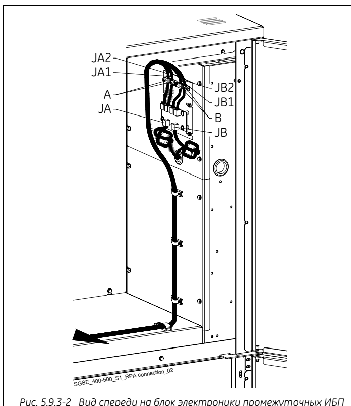
Рис. 5.9.3-2 Вид спереди на блок электроники промежуточных ИБП
