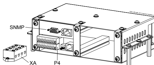
Рис. 2.1-4 Коммуникационный блок
