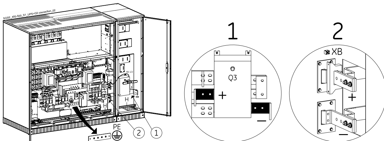
Рис. 10.5.1-3 Подключение опционального "Выключателя батарей Q3 в дополнительном шкафу"
