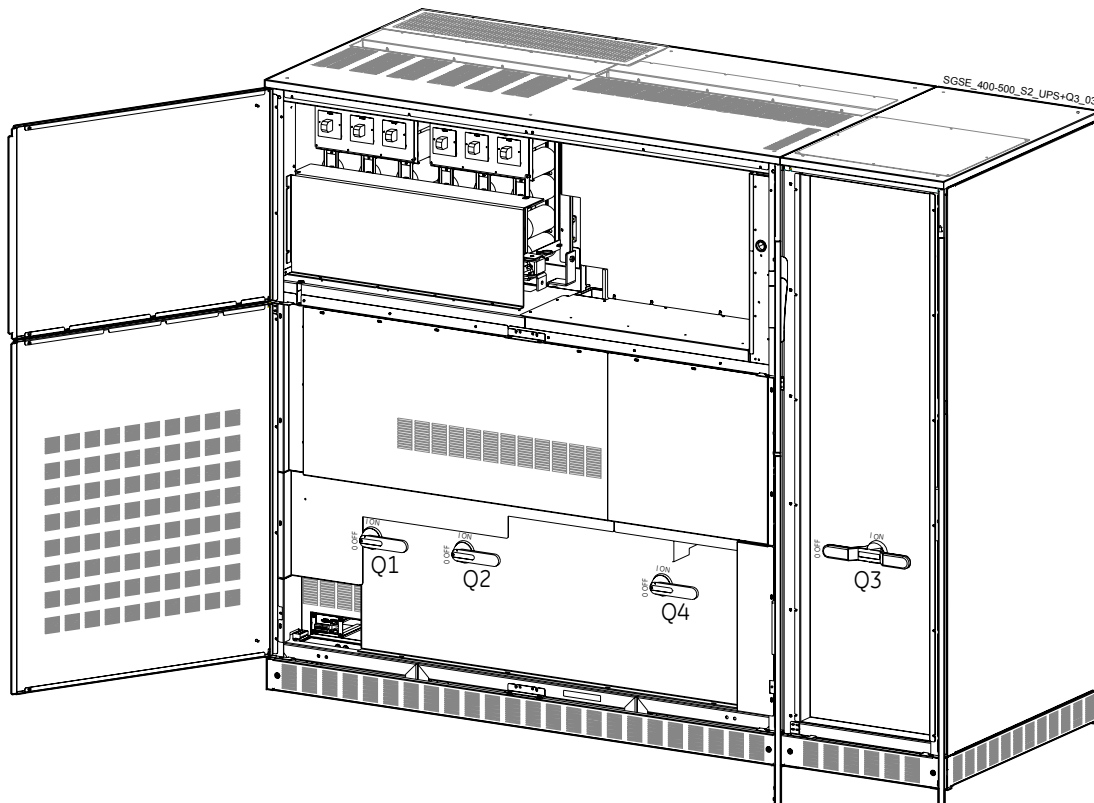
Рис. 2.2-2 Общий вид с открытыми дверями
