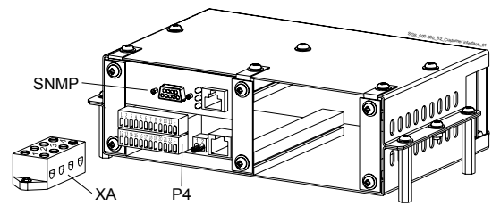
Рис. 2.2-4 Коммуникационный блок
