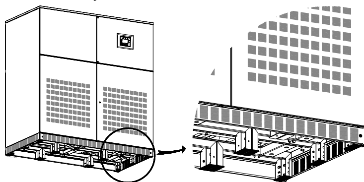
Рис. 5.4.1-4 Крепление шкафа ИБП к полу
