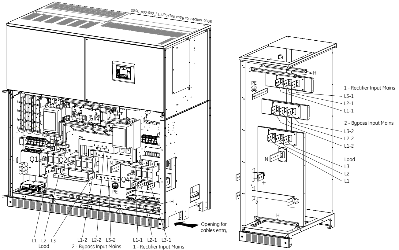
Рис. 10.5.2-3 Подключение
