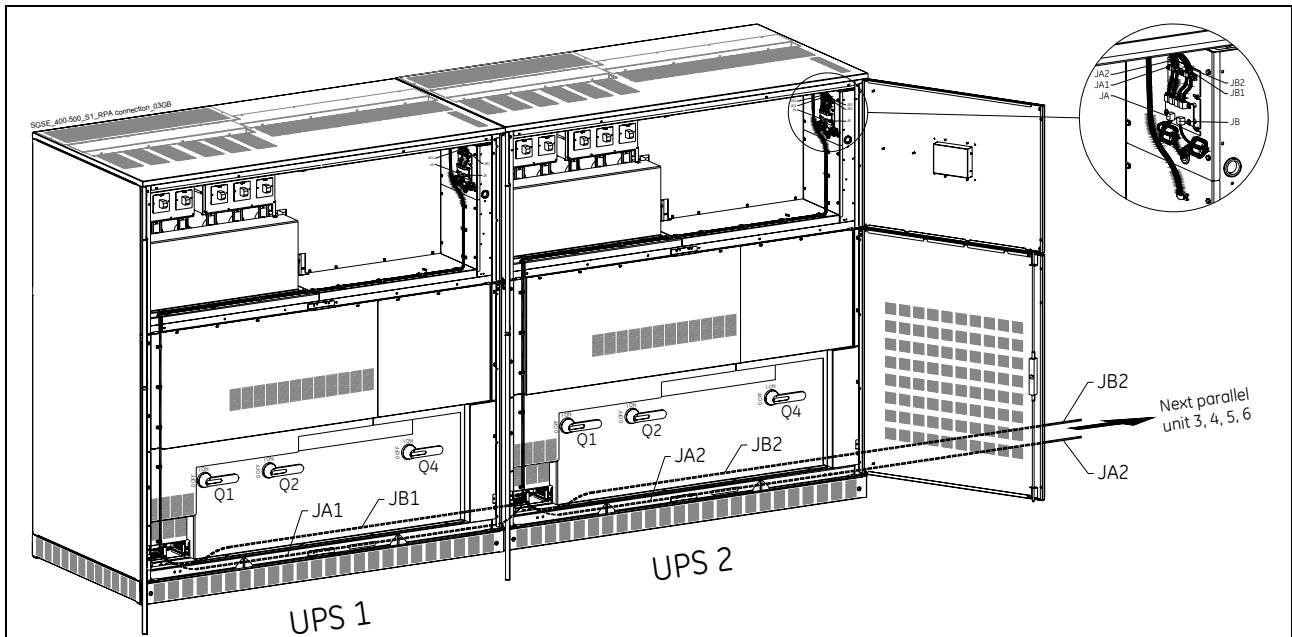
Рис. 5.9.3-3 Прокладка кабелей шины управления
