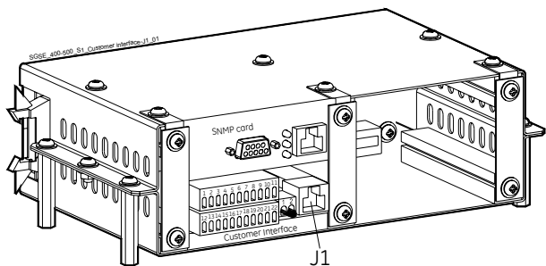
Рис. 9.1.1-1 RJ45 – место расположения розетки
