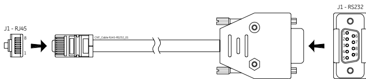
Рис. 9.1.1-2 RJ45 –RS232 переходной кабель
