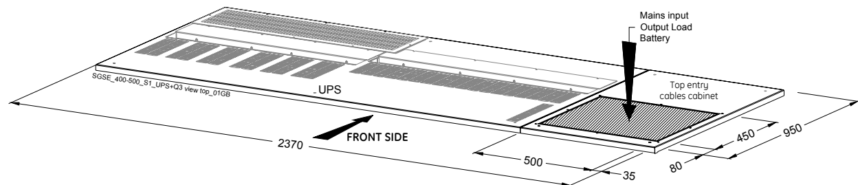
Рис. 5.4.1-4 ИБП SG-CE Series 400 – 500 кВА PurePulse® с шкафом выключателя АКБ Q3 и/или ввода кабелей сверху (опции)
